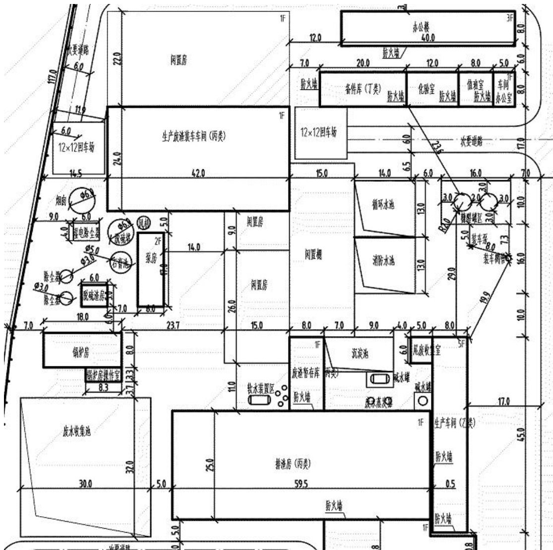
图2.2-3 平面布置图局部区域-区域二
